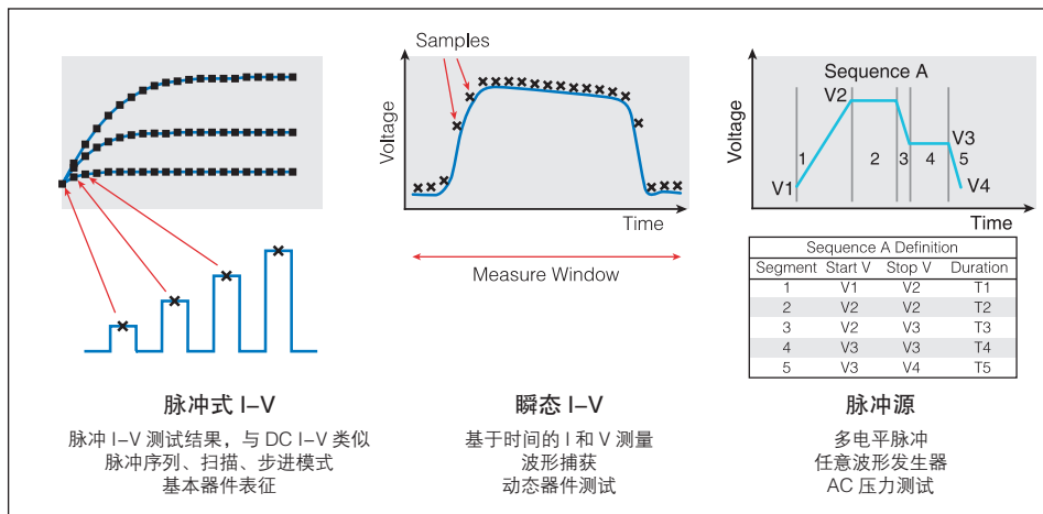
使用超快速脉冲式 I-V 最大限度地减少自热效应。
