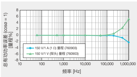
频率-功率精度特性示例
