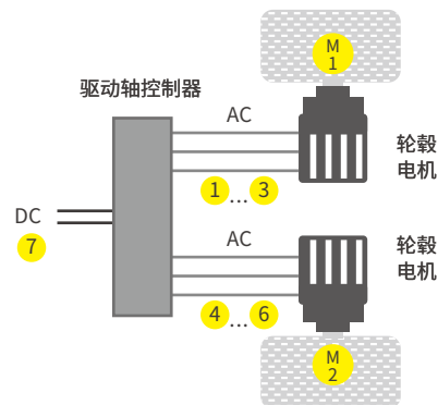
案例2: 车桥功率效率测量示例，从直流测量值(7)到双三相交流电测量值(1~3和4~6)以及双机械功率测量值(M1和M2)。
