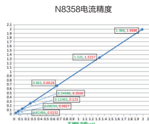
▲ 电流精度对比
