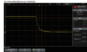
▲ N83624满载下降时间 (30.3 μs)
