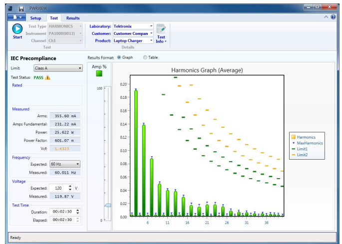
IEC 61000-3-2 电流谐波测试
