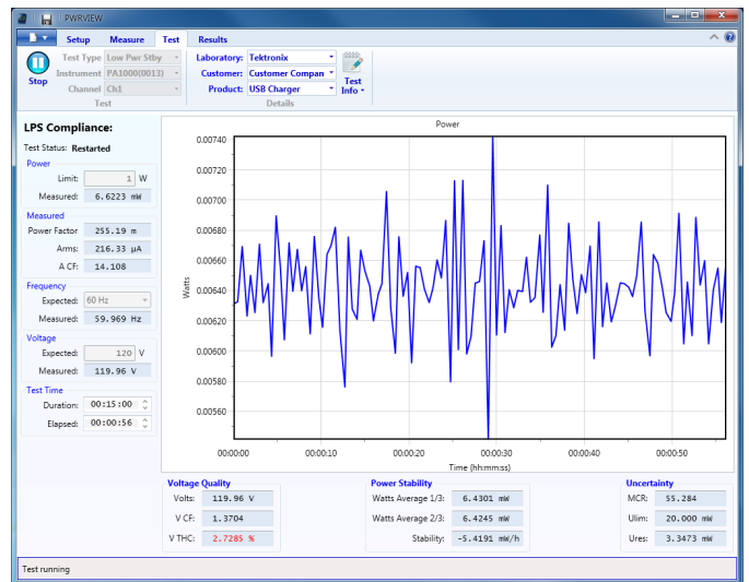
利用实时不确定性和稳定性测量进行 IEC 62301 备用电源测试
