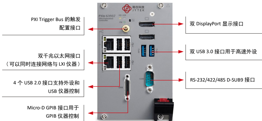
PXle-63937 前面板
