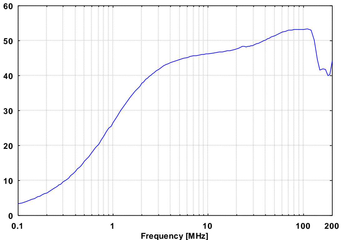
Impedanz an den Prüflingsklemmen (Kalibrieradapter KA 8126 F HYB erforderlich), BNC mit 50 \Omega Abschluss, Speiseklemmen kurzgeschlossen Impedance at EuT-Terminals (Calibration Adapter KA 8126 F HYB required), BNC-Port terminated with 50 \Omega , mains terminals shorted
